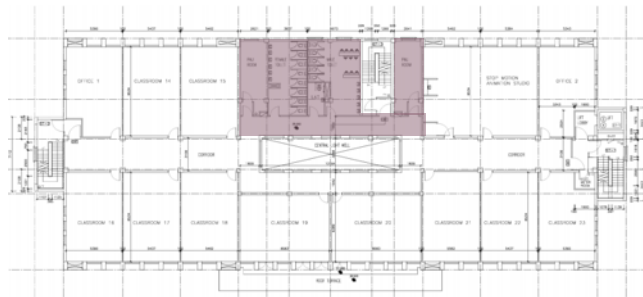
4/F Plan
